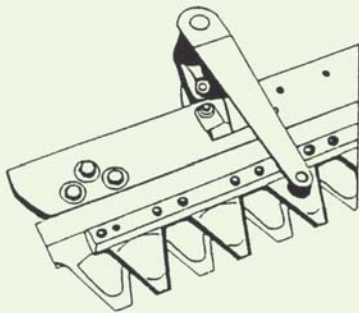
Doppel-Messerbalken
